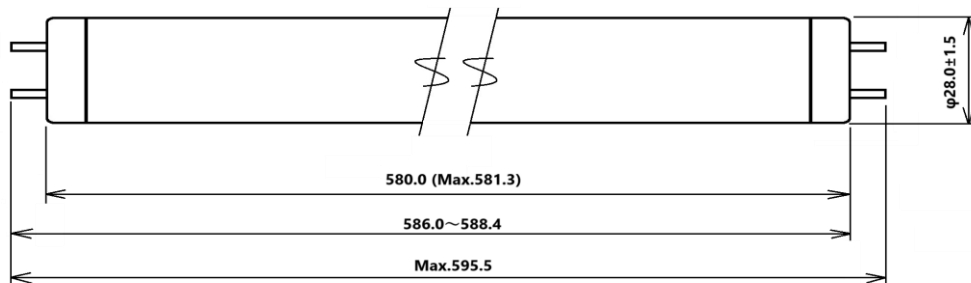
図－1 (単位:mm)
