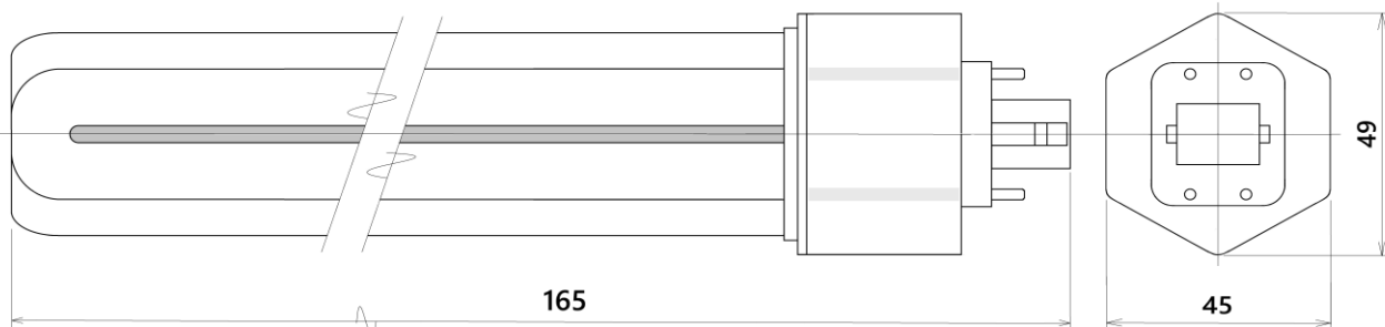
図-1 (単位:mm)
