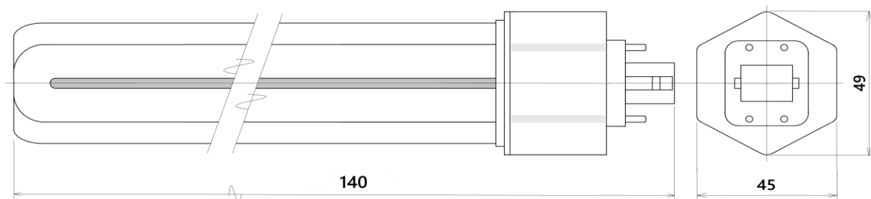
図-1 (単位:mm)
