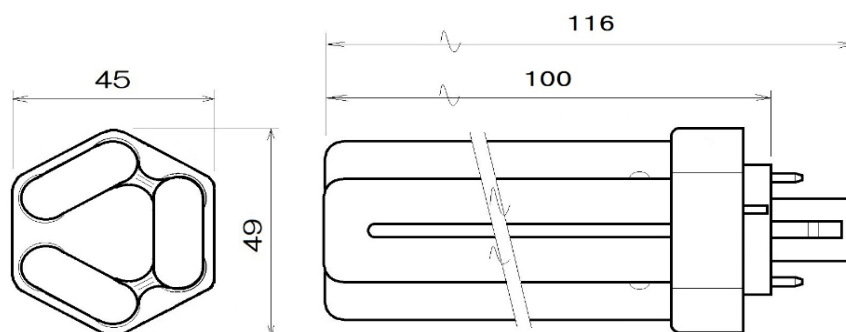
図-1 (単位:mm)
