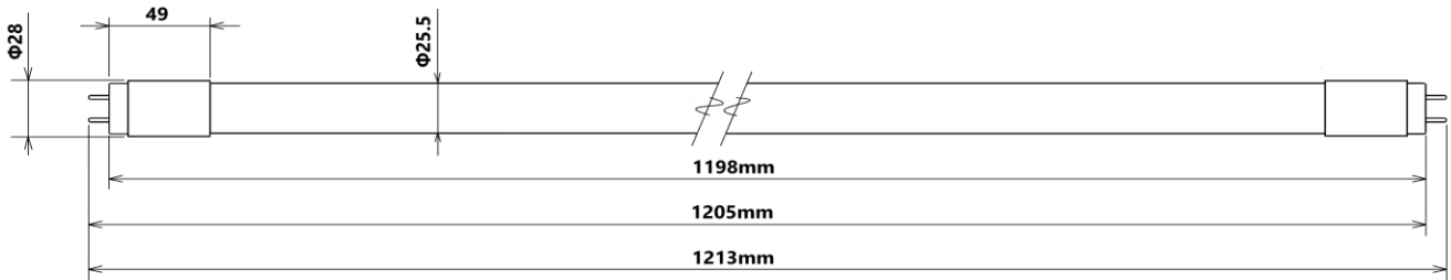
図－1 (単位:mm)
